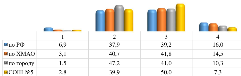
Распределение отметок по биологии
