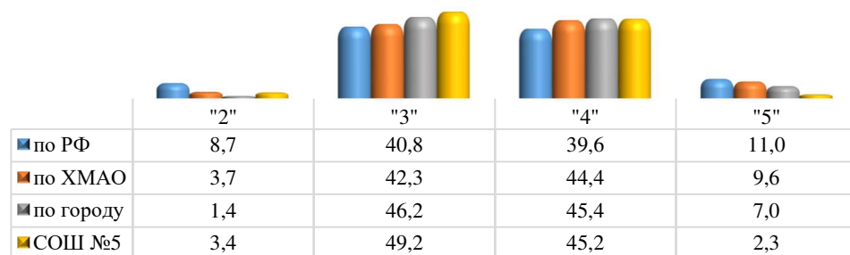
Распределение отметок по биологии
